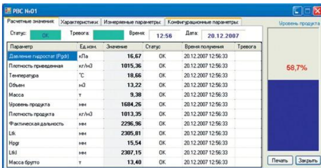
Рисунок 4 – Окно резервуара
