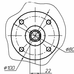
Рисунок В.1 – Габаритные и установочные размеры датчиков РДУЗ (лист 2)
