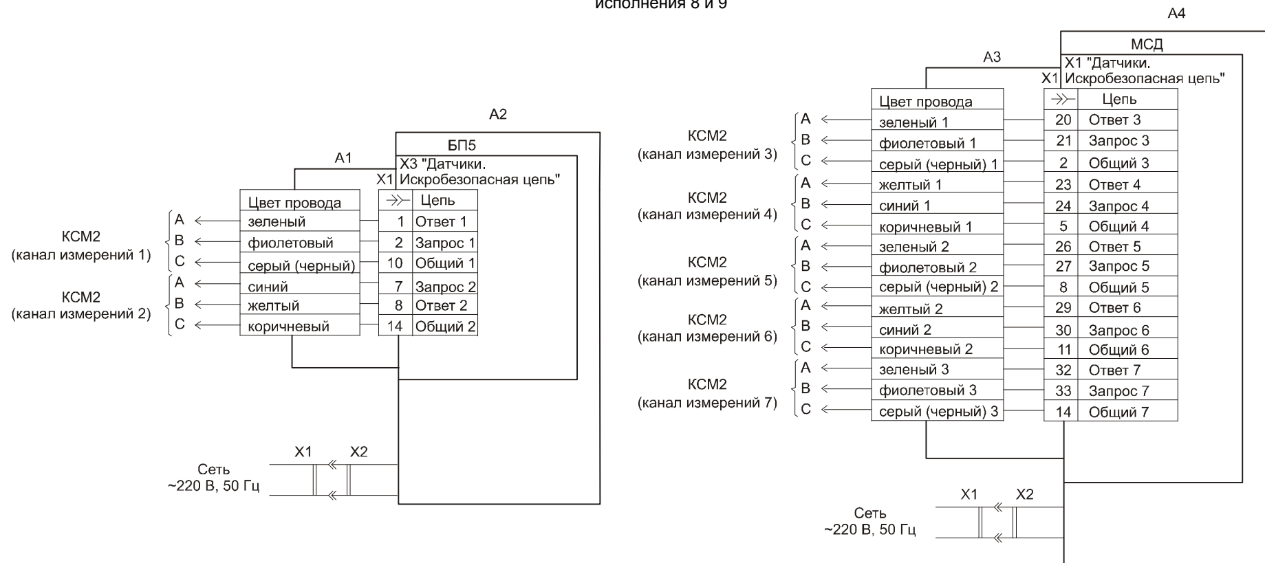
Рисунок G.3 – Схема соответствия выходных цепей контроллера KCM2 входным цепям контроллера микропроцессорного ГАММА-7/ГАММА-7М
