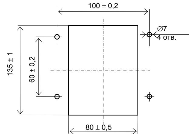
Рисунок 4 – Рекомендуемое посадочное место для установки прибора
