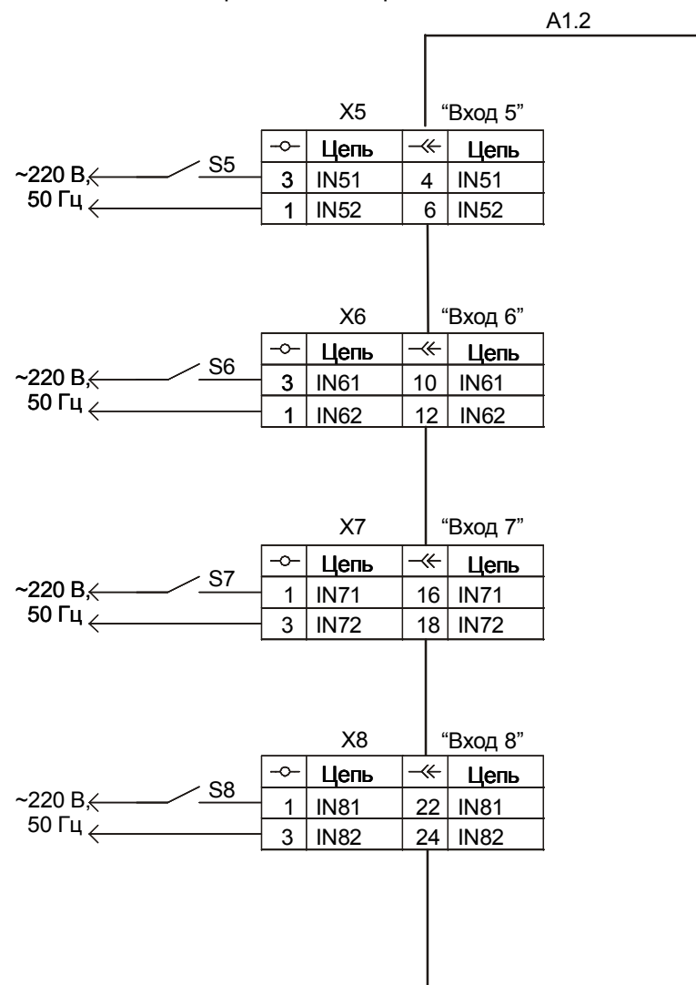
Рисунок А.8 – Схема подключения МВЗ (лист 2)
