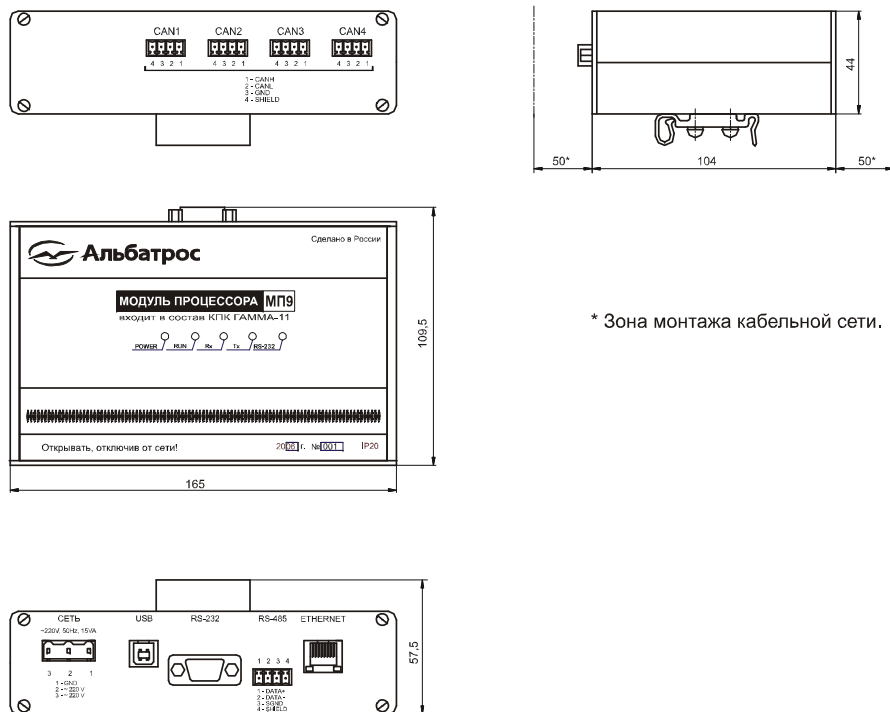
Рисунок 6 – Внешний вид и габаритные размеры МП9
