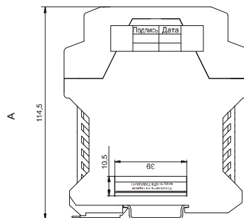
Рисунок 4 – Внешний вид и габаритные размеры составных частей прибора (вариант установки модулей прибора на один DIN-рельс, повернуто)
