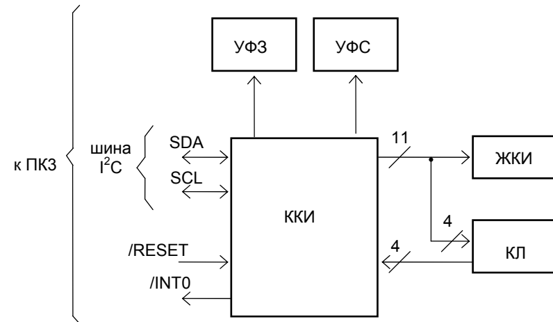
Рисунок 3 – Структурная схема ячейки индикации ЯИ14
