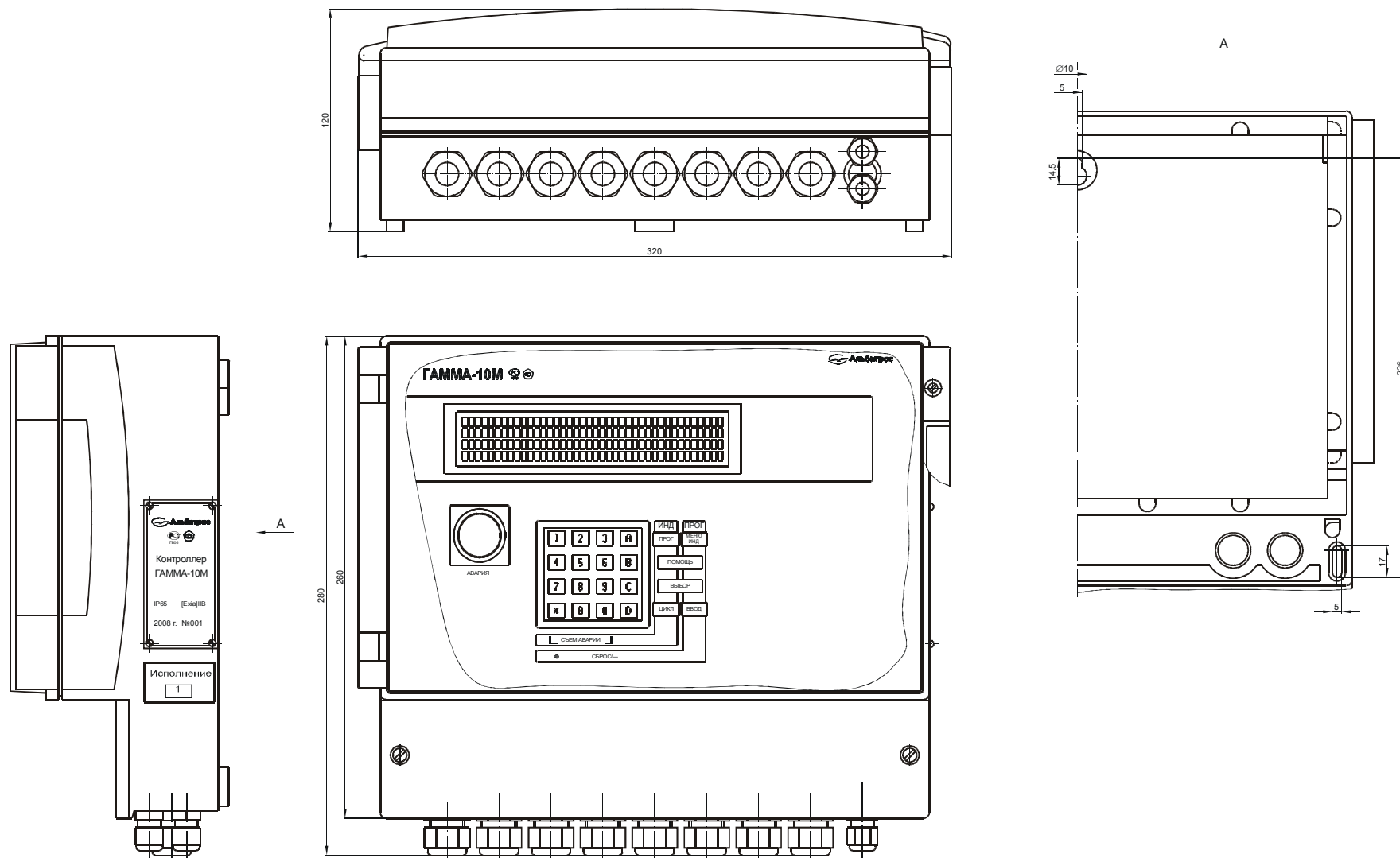
Рисунок 1 – Внешний вид и габаритные размеры прибора
