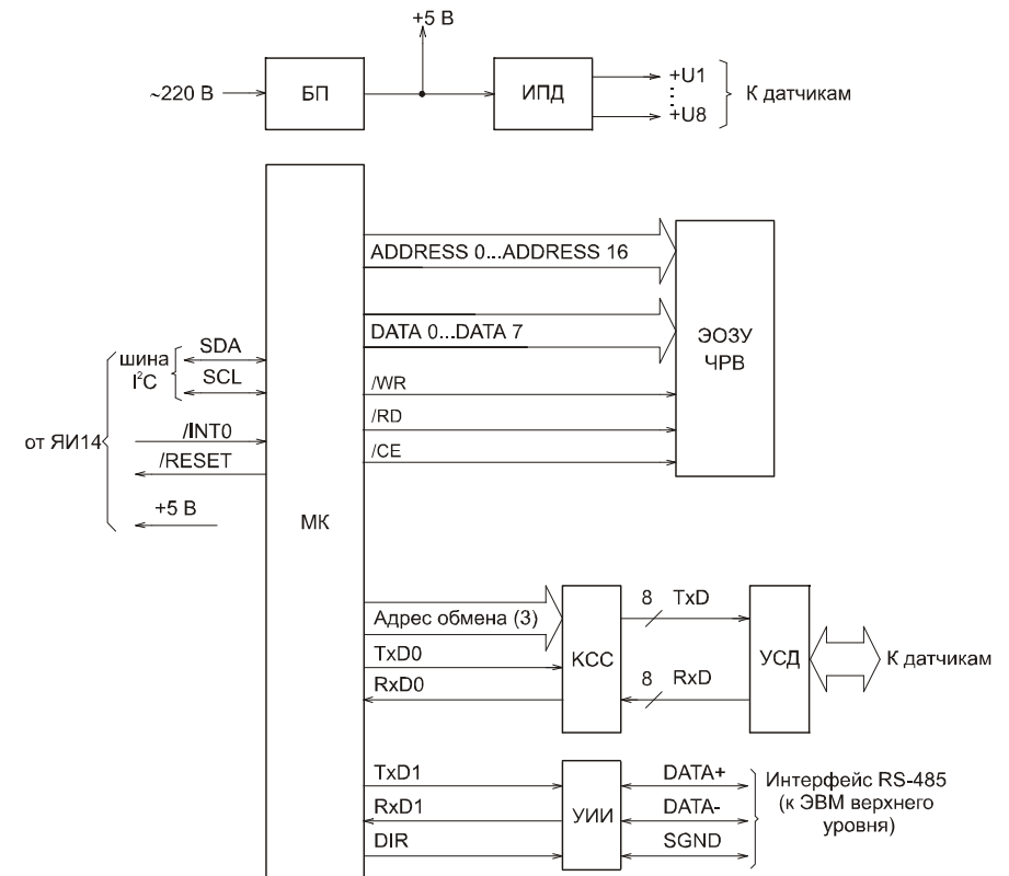
Рисунок 2 – Структурная схема платы коммутации ПКЗ
