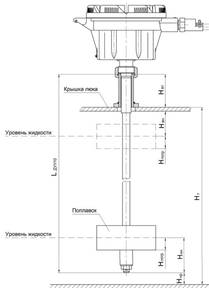
Рисунок 1 - Схема определения длины ЧЭ уровнемеров с поплавком типа I
