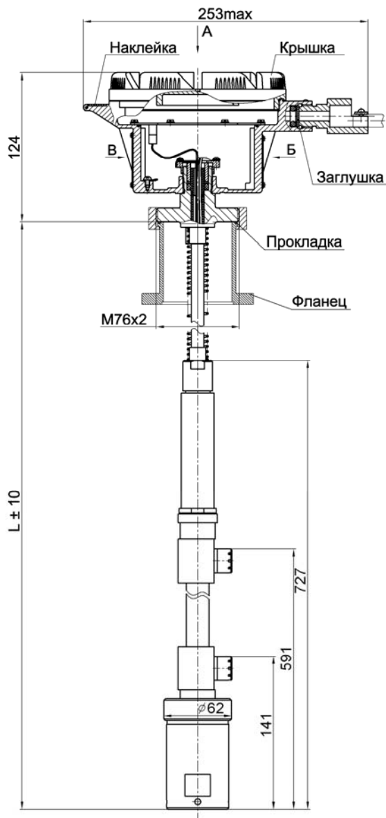
Внешний вид, схема определения длины ЧЭ и высоты установки плотномера
